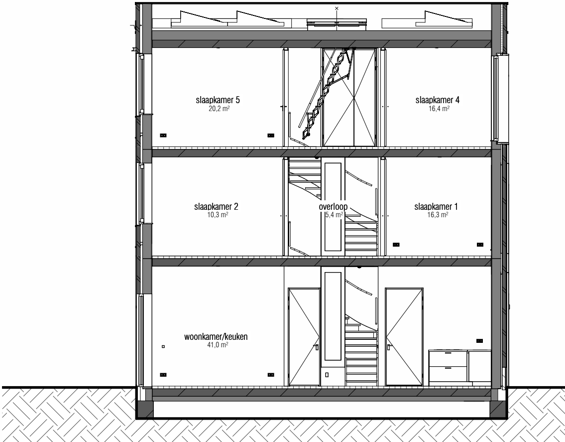
doorsnede 1 : 100
