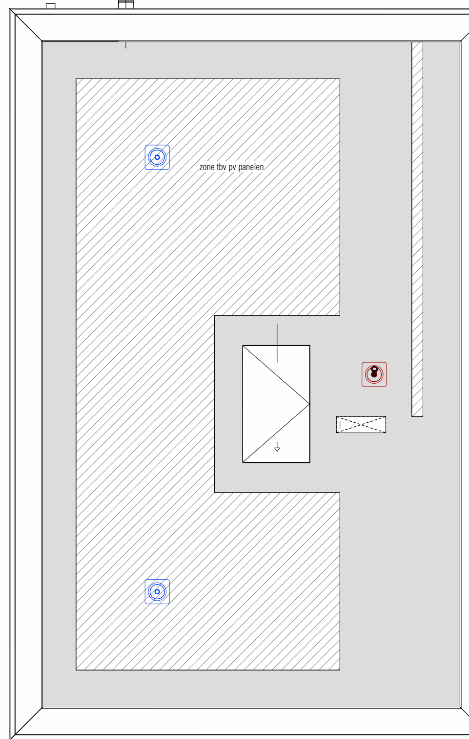
dak verdieping 1 : 50
