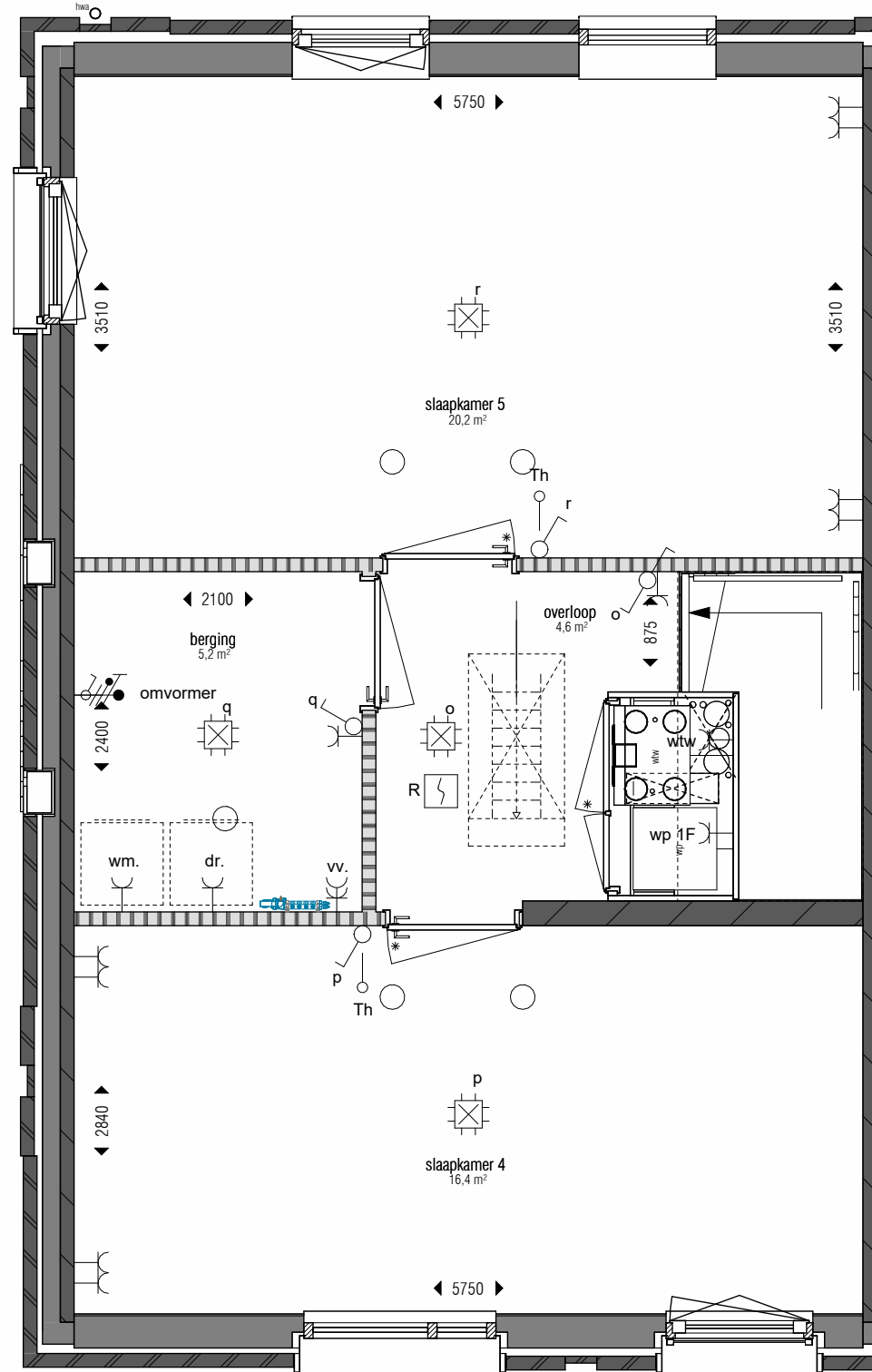
tweede verdieping 1 : 50
