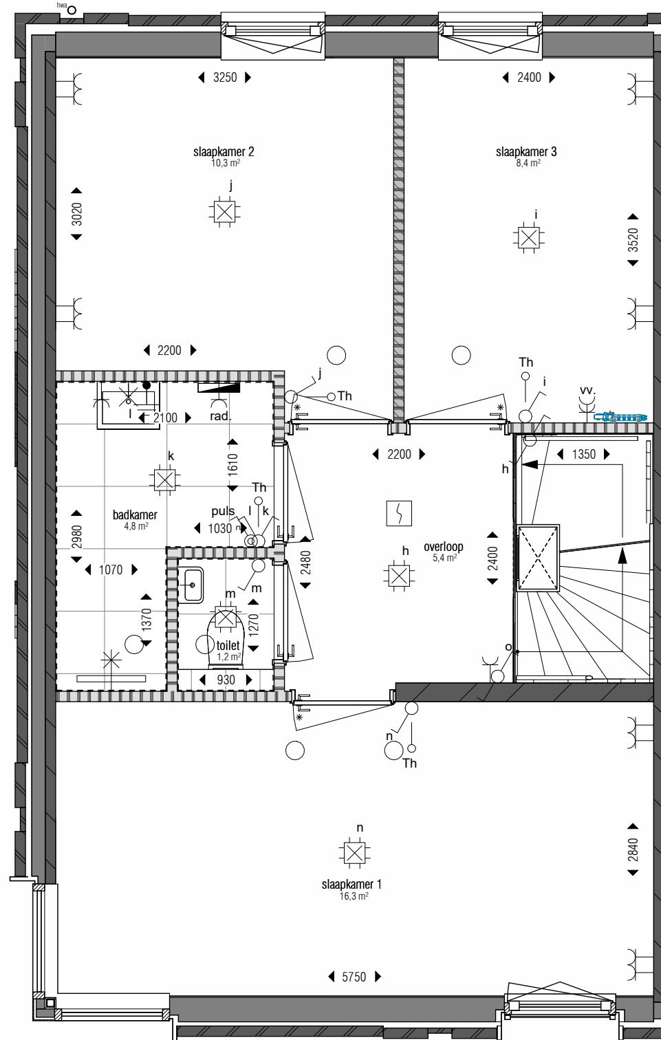
eerste verdieping 1 : 50
