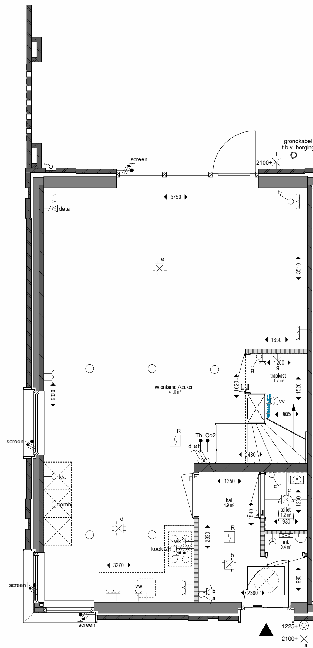
begane grond 1 : 50
