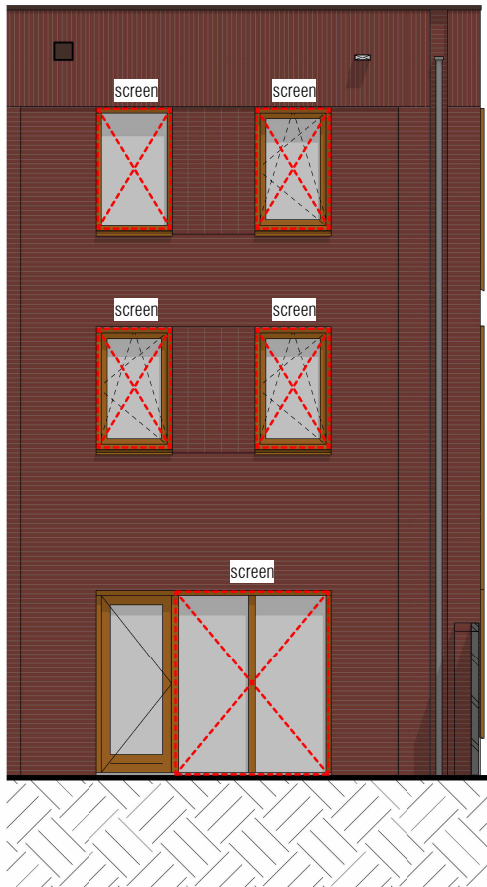
achtergevel 1 : 100
